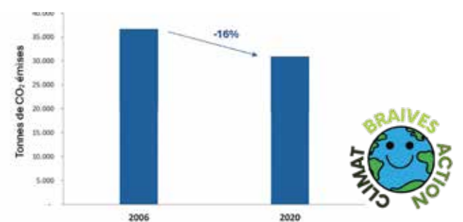
Evolution des émissions de CO 2 sur la commune de Braives de 2006 à 2020 : -16%
